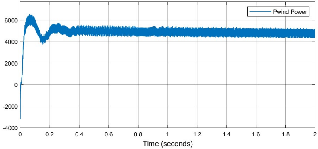
Fig 8: WindPowerVsTimeWaveform
