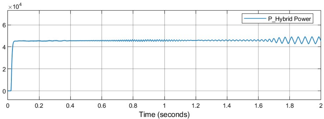
Fig 10: HybridSystemtotalpowerVsTimeWaveform
