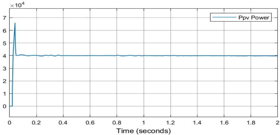
Fig 7: PVPowerVsTimeWaveform
